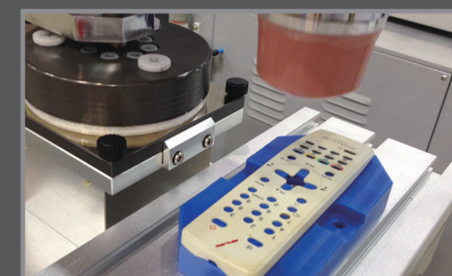
移印机 Pad Printer
